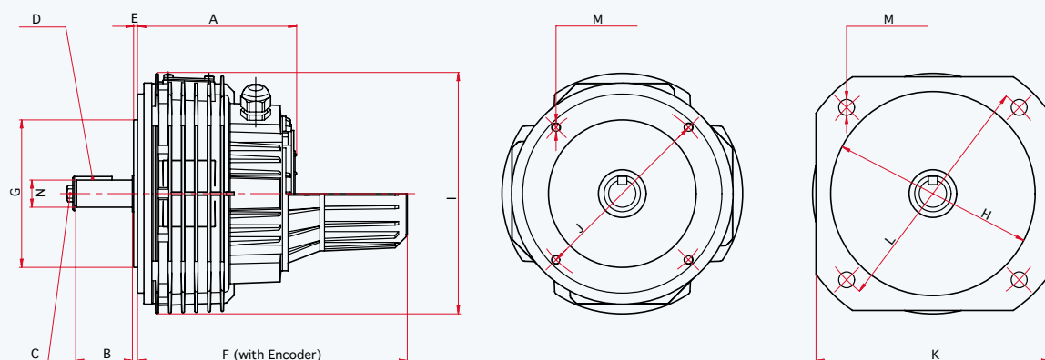
FLANGE B-14
