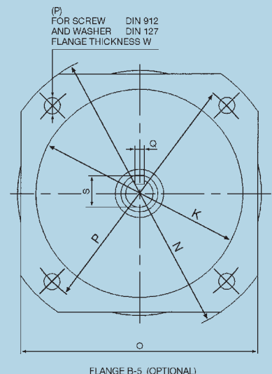
FLANGE B-5 (OPTIONAL)
