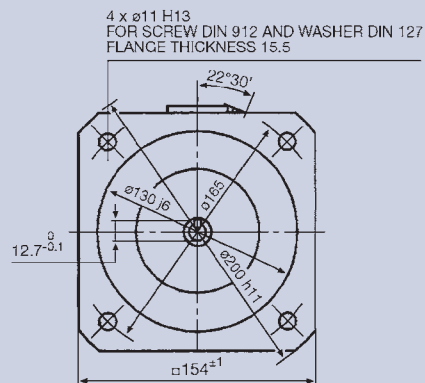
FLANGE B-5 (OPTIONAL)
