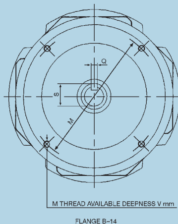
FLANGE B-14
